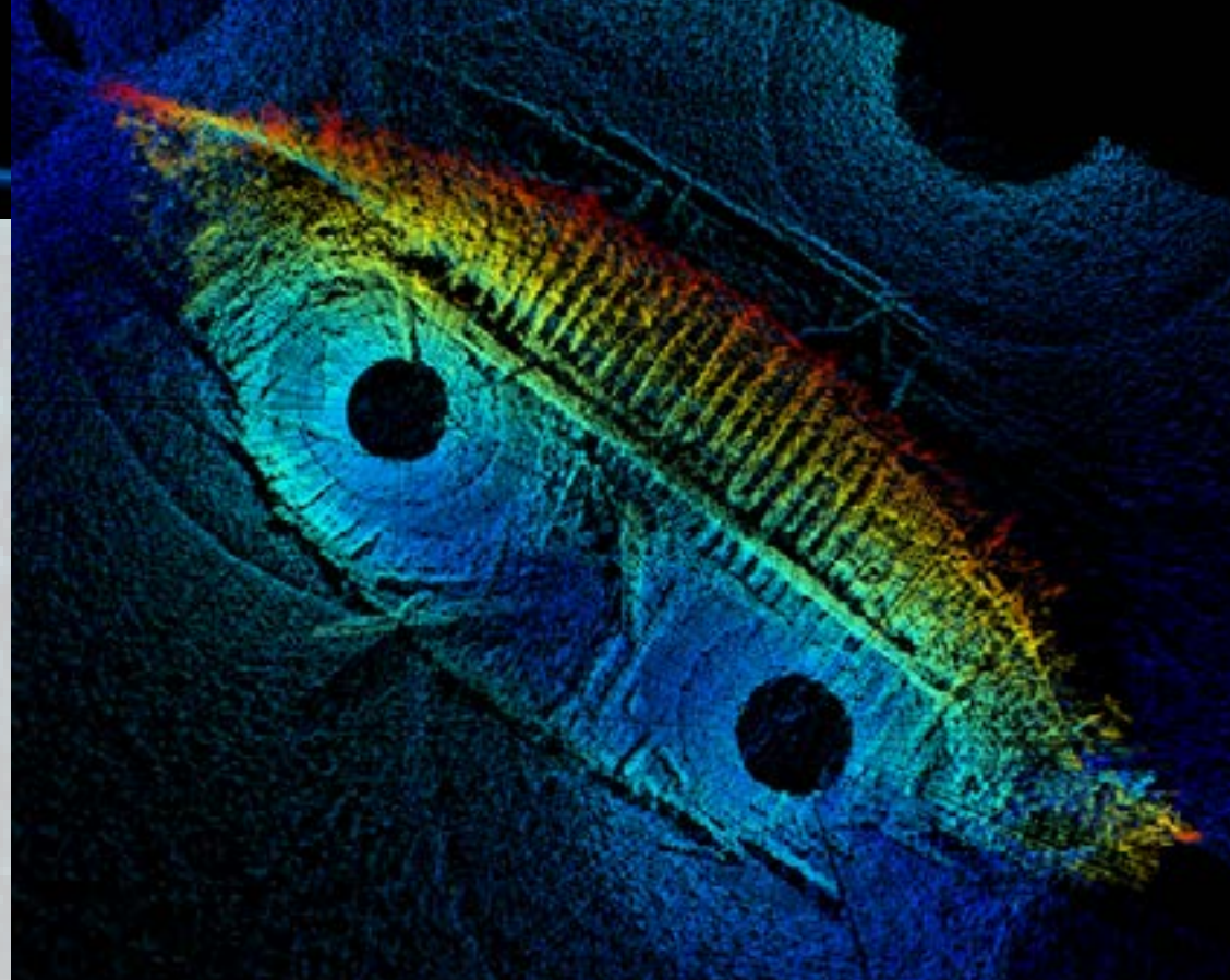
3D-punktmoln, data sammanfogat av sju separata scannningar, de svarta ringarna är där scannern har sått.
